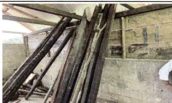
Foto 5: Vigas de madera destruidas.
